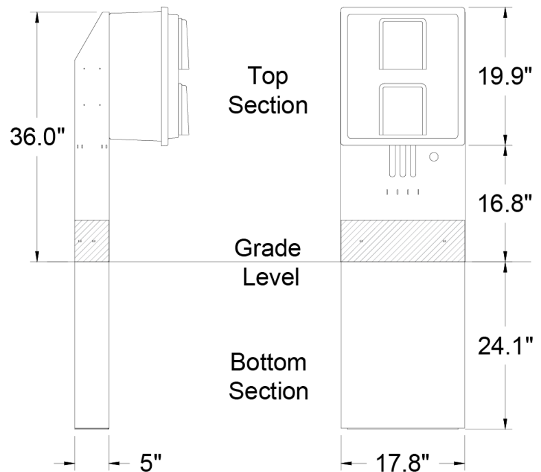
Actual Dimensions Shown Here
